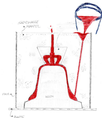
Schematische Darstellung des Glockengusses
